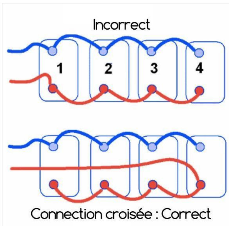
Connection croisée (max 4 batteries en parallèle)
